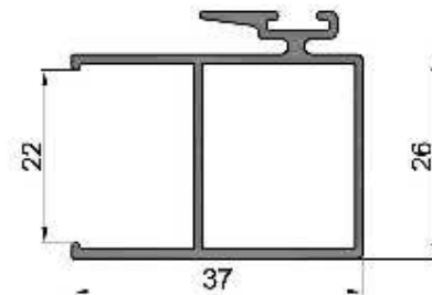
LM-250 (MBM 4234) Parante Central DVH Peso: 0,553 kg/ml Paquete x 6 tiras
