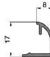
LM-233 (MBM 4309) Contravidrio curvo 8mm Peso: 0,135 kg/ml Paquete x 12 tiras
