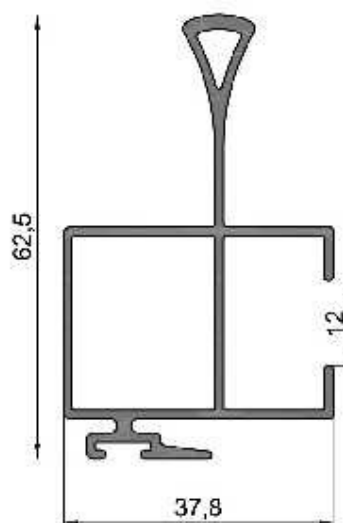
LM-208 (MBM 4344) Parante central con Tirador Peso: 0,772 kg/ml Paquete x 2 tiras
