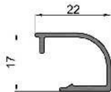
LM-232 (MBM 4310) Contravidrio curvo 22mm Peso: 0,202 kg/ml Paquete x 12 tiras
