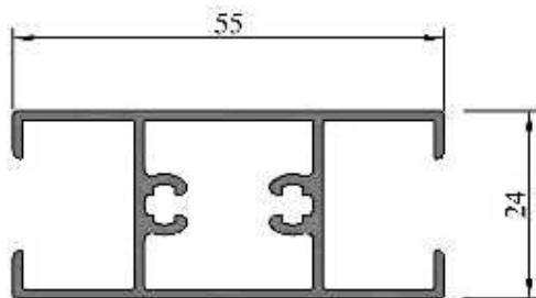
LM-239 (MBM 4239) Travesaño hoja vidrio simple puerta corrediza Peso: 0,660 kg/ml
