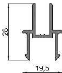
LM-246 (MBM 4324) Encuentro central de 4 hojas ventana y puerta corrediza Peso: 0,285 kg/ml
