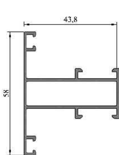
LM-221 (MBM 4221) Travesaño angosto pañó fijo Peso: 0,728 kg/ml
