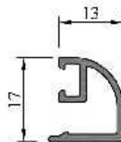
LM-237 (MBM 4237) Contravidrio curvo Portafelpa Peso: 0,180 kg/ml Paquete x 12 tiras
