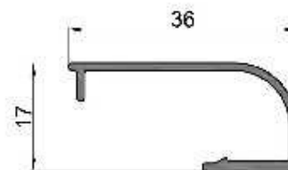
LM-257 (MBM 4314) Contravidrio curvo 36mm Peso: 0,254 kg/ml Paquete x 12 tiras
