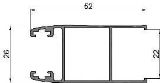
LM-248 (MBM 4233) Parante Lateral DVH Peso: 0,580 kg/ml Paquete x 6 tiras
