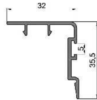
LM-907 (MBM 4260) Complemento Parante Central 45° Peso: 0,338 kg/ml
