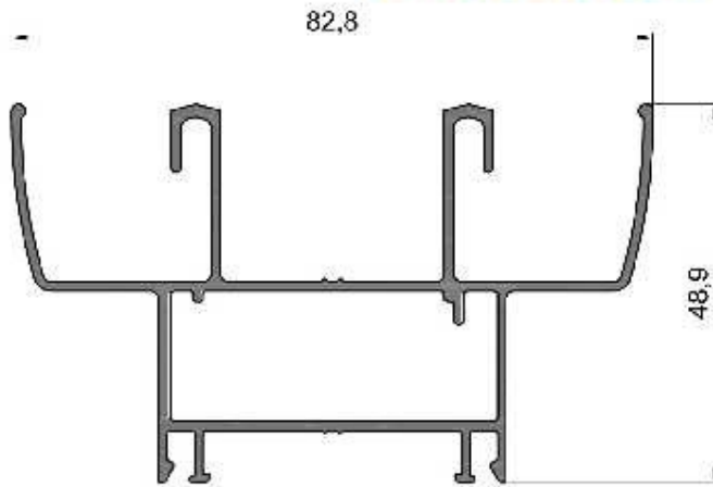
LM-906 (MBM 4259) Marco Perimetral Corrediza 45° Peso: 1,100 kg/ml
