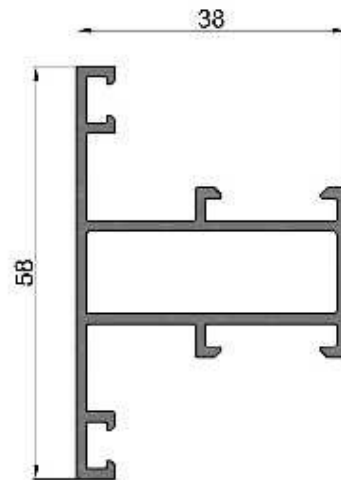
LM-264 (MBM 4330) Travesaño para paño fijo curvo Peso: 0,680 kg/ml
