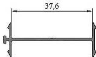
LM-213 (MBM 4216) Acople marco Peso: 0,244 kg/ml
