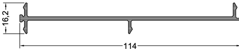
499346 0.708 Kg/m ACOPLE 180°
