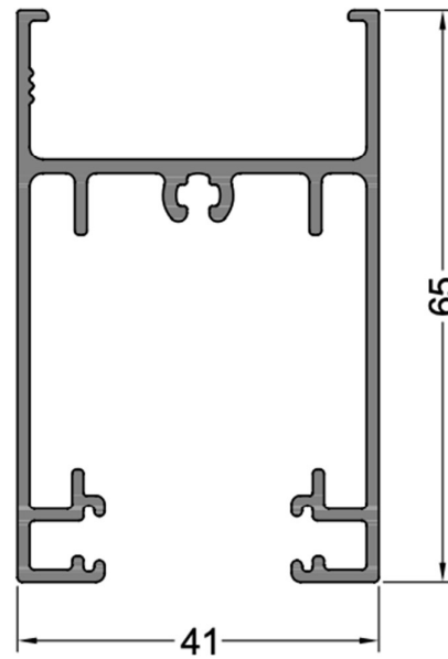
4261 0.955 Kg/m CORREDIZA HOJA DINTEL DVH
