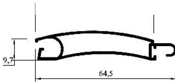
LH-307 (MPB 4249) Tablilla cortina de enrollar Peso: 0,420 kg/ml
