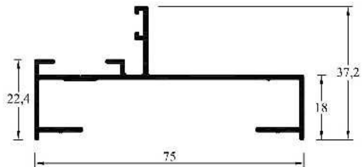
LH-031 (MPB 3789) Marco Postigón Grande Peso: 0,560 kg/ml Paquete x 6 tiras Peso aprox. paq.: 20,2 kg
