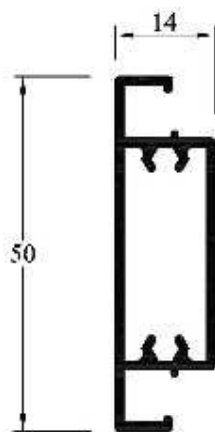
LH-090 (MPB 3647) Travesaño Hoja Mosquitero Peso: 0,460 kg/ml Paquetes x 8 tiras Peso aprox. paq.: 22,1 kg
