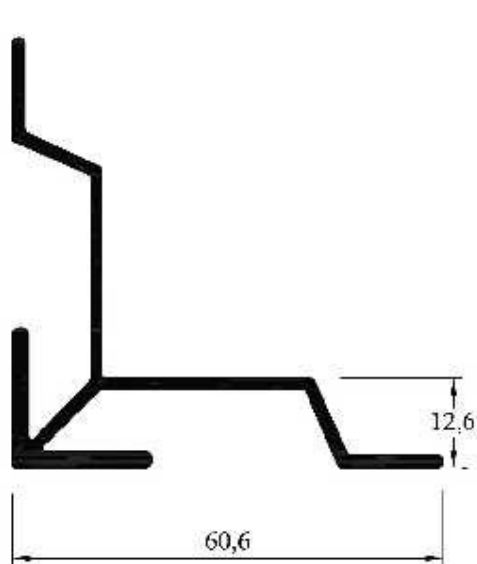
LH-016 (MPB 3749) Escuadra 13 mm Pesada Peso: 0,520kg/ml Paquete x 4 tiras Peso aprox. paq.: 12,5 kg
