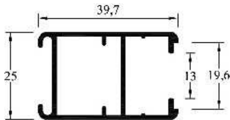
LH-028 (MPB 3785) Parante Chico Postigón Peso: 0,480 kg/ml Paquete x 8 tiras Peso aprox. paq.: 23,1 kg
