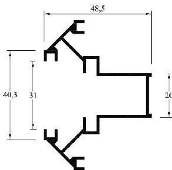
LH-051 (MPB 3527) Columna Tabique Peso: 0,710 kg/ml Paquete x 4 tiras Peso aprox. paq.: 17,1 kg
