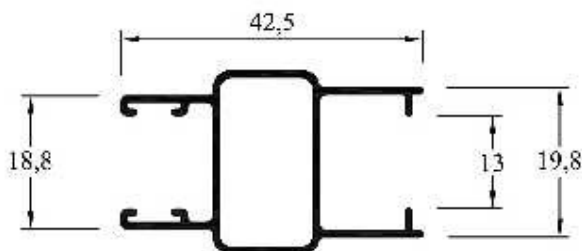
LH-103 (MPB 4103) Parante Lateral Chico Pcs: 0,365 kg/ml Paquete x 8 tiras Peso aprox. paq.: 17,7 kg
