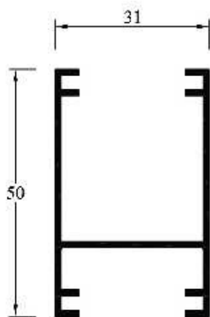
LH-049 (MPB 3526) Travesaño Tabique Peso: 0,560 kg/ml Paquete x 6 tiras Peso aprox. paq.: 20,2 kg
