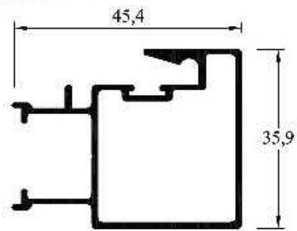
LH-154 (MPB 3939) Parante Central Reforzado Peso: 0,570 kg/ml Paquete x 6 tiras Peso aprox. paq.: 20,6 kg
