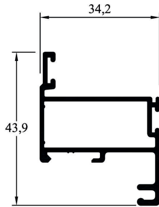
LH-071 (MPB 4243) Hoja Inferior Peso: 0,495kg/ml
