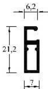
LH-009 (MPB 3650) Canal 9 Mosquitero Liviano Peso: 0,190 kg/ml Paquete x 20 tiras Peso aprox.paq.: 22,8 kg
