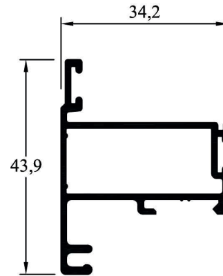
LH-072 (MPB 4244) Hoja Superior Peso: 0,495kg/ml
