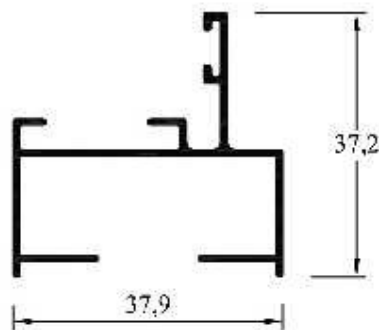
LH-030 (MPB 3900) Marco Chico Postigón Peso: 0,340 kg/ml Paquete x 10 tiras Peso aprox. paq.: 20,4 kg
