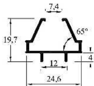
LH-018 (MPB 3761) Perimetral VRP Rayado Peso: 0,195 kg/ml Paquete x 15 tiras Peso aprox. paq.: 17,6 kg
