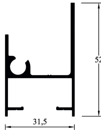
LH-070 (MPB 4242) Marco Chico Ventana Banderola Peso: 0,525 kg/ml
