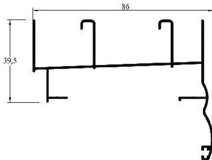
LH-067 (MPB 4251) Marco corrediza con contramarco Peso: 0,740 kg/ml
