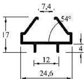
LH-022 (MPB 3394) Perimetral VRP Liso Chico Peso: 0,175 kg/ml Paquete x 15 tiras Peso aprox. paq.: 15,8 kg
