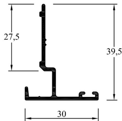
LH-945 (MPB 4481) Encuentro de hoja 36 mm Peso: 0,297 kg/ml Paquete x 10 tiras Peso aprox. paq.: 18 kg
