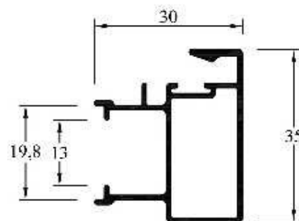
LH-004 (MPB 3549) Parante Central Grande Peso: 0,425 kg/ml Paquete x 8 tiras Peso aprox. paq.: 20,5 kg
