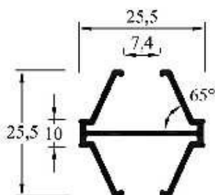
LH-020 (MPB 3762) Nudo VRC(sin Cava) Peso: 0,250 kg/ml Paquete x 10 tiras Peso aprox. paq.: 15,1 kg
