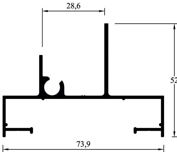
LH-069 (MPB 4241) Marco Ventana Banderola Peso: 0,735 kg/ml
