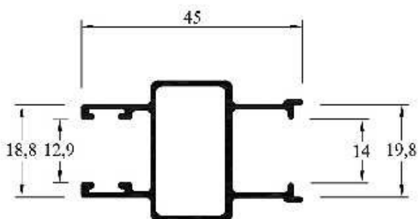
LH-003 (MPB 3546) Parante Lateral Grande Peso: 0,425kg/ml Paquete x 8 tiras Peso aprox. paq.: 20,5 kg
