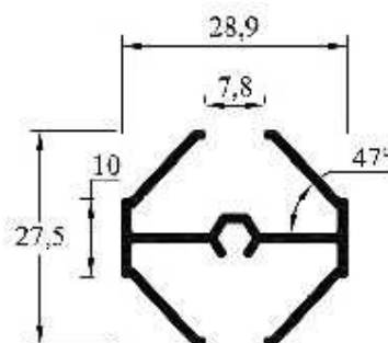
LII-026 (MPB 3503) Nudo VRC Gde (con Cava) Peso: 0,330 kg/ml Paquete x 10 tiras Peso aprox. paq.: 19,8 kg
