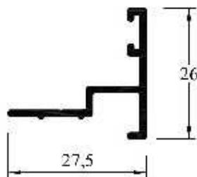
LH-030 (MPB 3900) Marco Chico Postigón Peso: 0,340 kg/ml Paquete x 10 tiras Peso aprox. paq.: 20,4 kg
