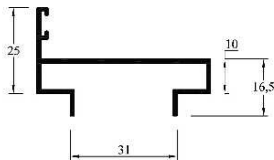
LH-052 (MPB 3811) Marco Puerta Placa Peso: 0,400 kg/ml Paquete x 4 tiras Peso aprox. paq.: 9,6 kg
