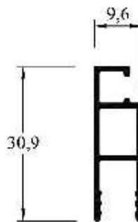
LH-005 (MPB 3708) Hoja Mosquitero Peso: 0,320 kg/ml Paquete x 10 tiras Peso aprox.paq.: 19,2 kg
