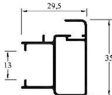
LH-104 (MPB 4104) Parante Central Chico Peso: 0,350 kg/ml Paquete x 8 tiras Peso aprox. paq.: 16,9 kg
