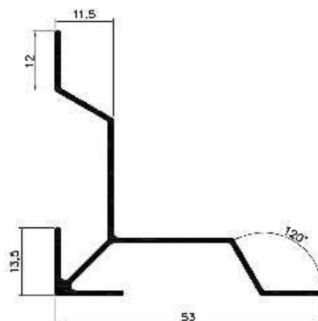
LH-159 (MPB 4348) Escuadra reforzada Peso: 0,480 kg/ml Paquete x 6 tiras Peso aprox. paq.: 17,3 kg
