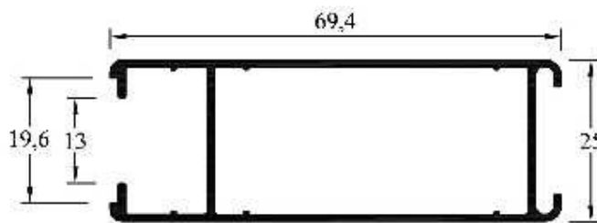
LH-029 (MPB 3823) Parante Grande Postigón Peso: 0,590 kg/ml Paquete x 4 tiras Peso aprox. paq.: 13,7 kg
