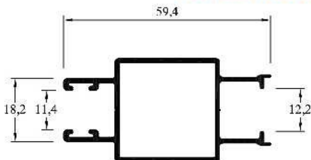
LH-153 (MPB 3938) Parante Lateral Reforzado Peso: 0,621 kg/ml Paquete x 6 tiras Peso aprox. paq.: 22,4 Kg
