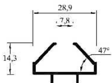
LH-025 (MPB 3502) Marcos VRP Liso Gde Peso: 0,215 kg/ml Paquete x 15 Tiras Peso aprox. paq.: 19,4 kg
