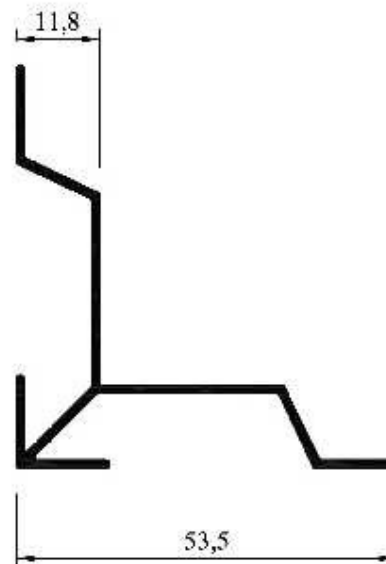
LH-027 (MPB 3752) Escuadra 2001 Liviana Peso: 0,350 kg/ml Paquete x 6 tiras Peso aprox. paq.: 12,6 kg
