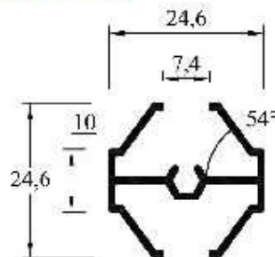
LH-023 (MPB 3943) Nudo VRC Liso Chico (con Cava) Peso: 0,260 kg/ml Paquete x 10 tiras Peso aprox. paq.: 15,8 kg
